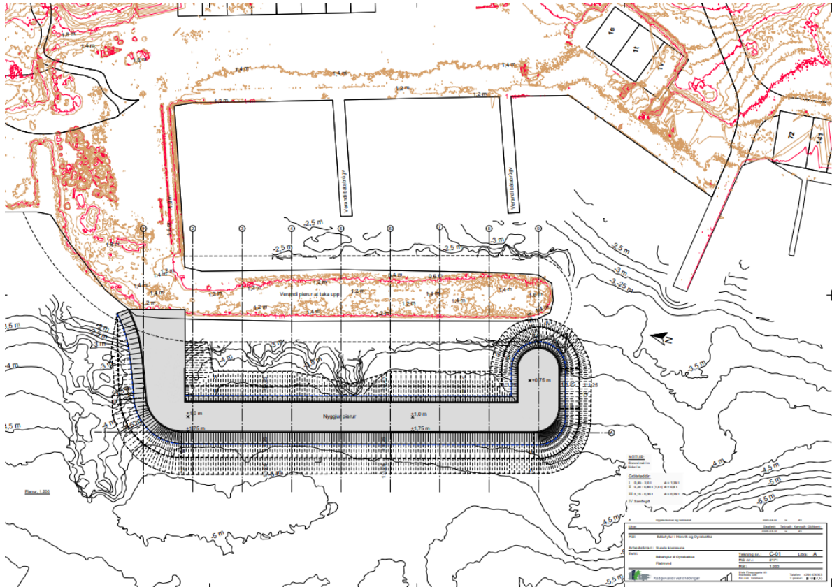
Mynd 2 Flatmynd av nýggja pirinum, sum ætlanin er at gera í bátahylinum á Oyrarbakka (tekning C-01)
