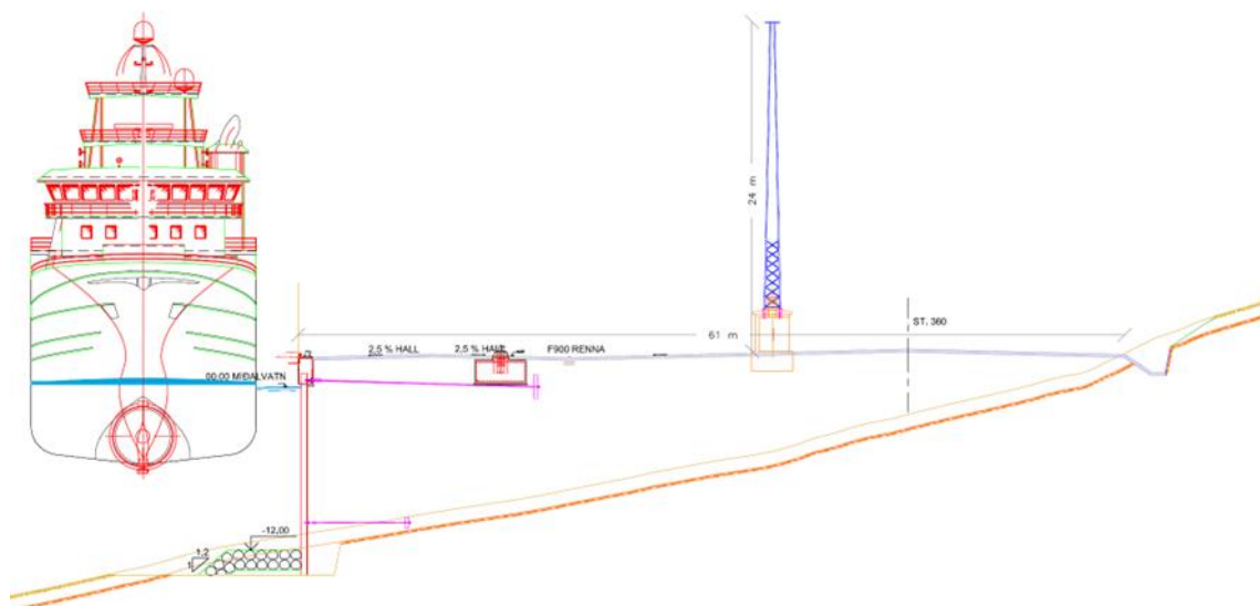
Mynd 3. Prinsippvørskurður av bryggjuni Undir Gøtueiði
