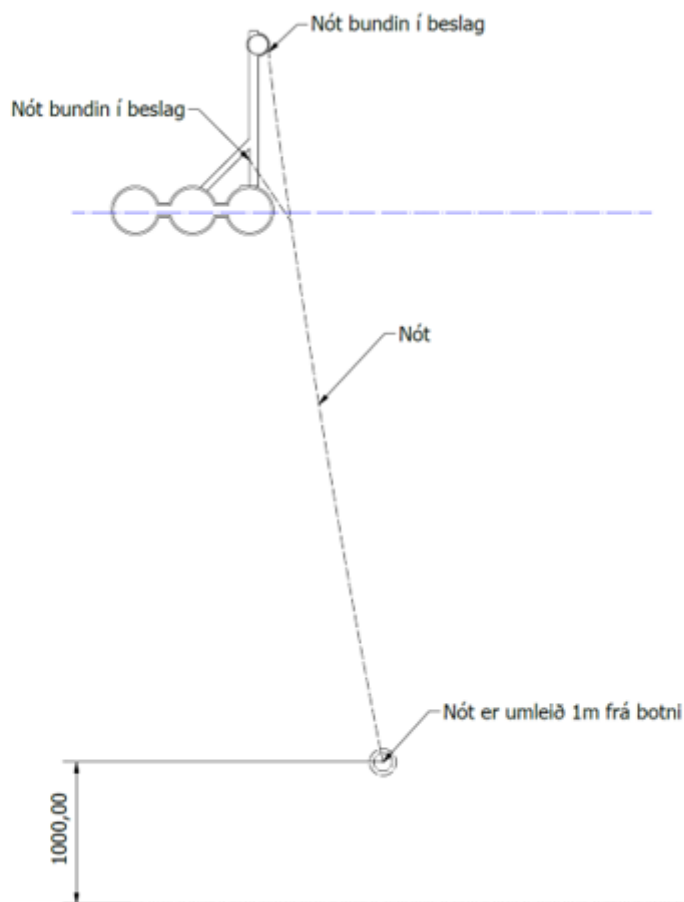
Mynd 4. Tekning av flótisþerru, ið skal forða fyri, at plast sleppur út í umhvørvið.
