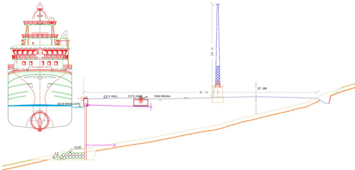
Mynd 5. Prinsippvørskurður av kaiini.
