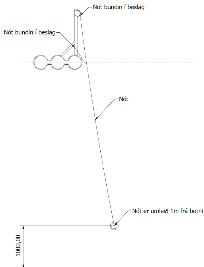
Mynd 17. Tvørskurður av flótisperru.
