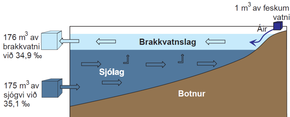
Mynd 11. Lýsing av lagdeilingini á fjørðinum
