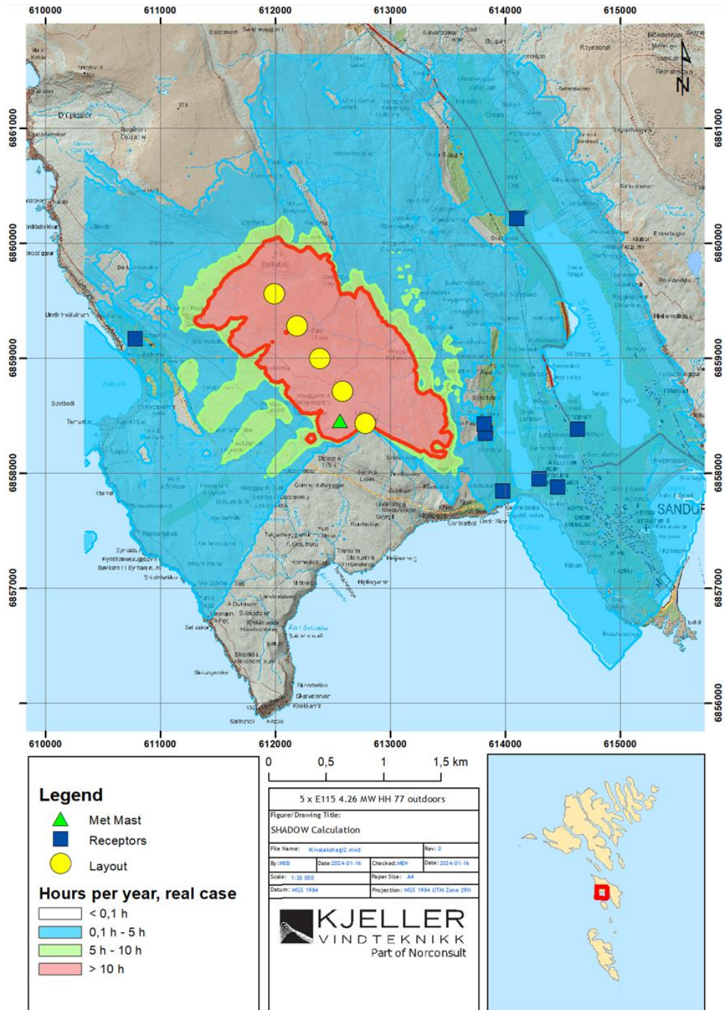
Mynd 2 Skuggakast fyr 5 x E115 á 4,26 MW HH 77 m
