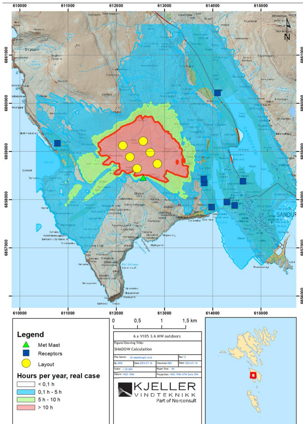
Mynd 1 Skuggakast fyri 6 x V105 á 3,6 MW
