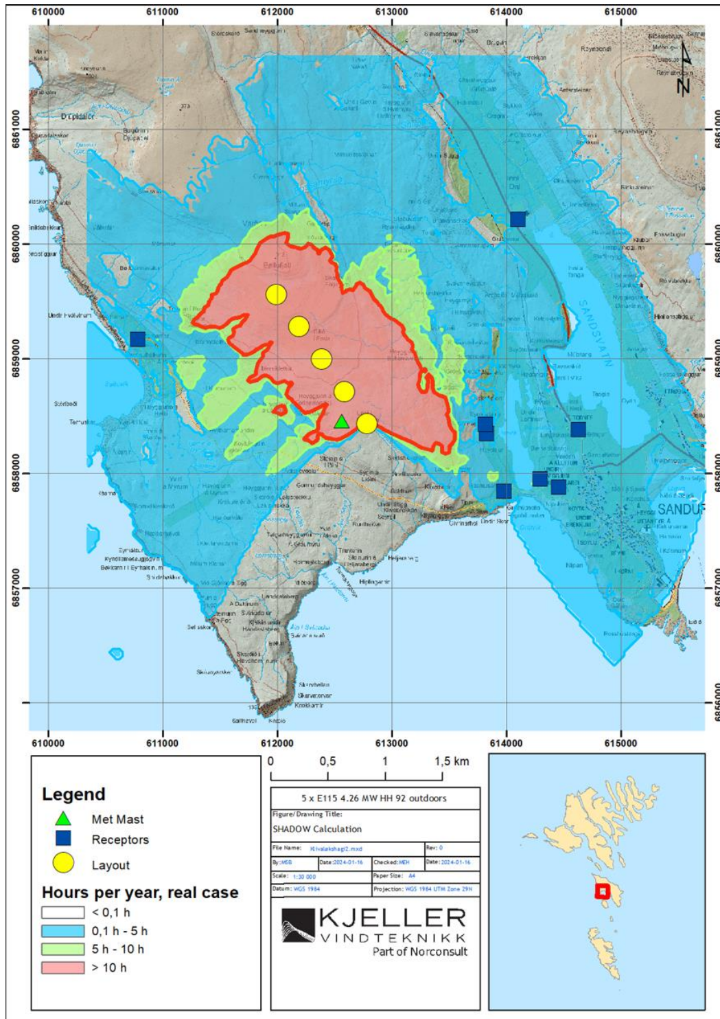
Mynd 3 Skuggakast fyrir 5 x E115 á 4,26 MW HH 92 m
